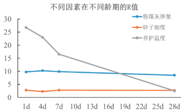
图4 不同因素在不同龄期的R值
