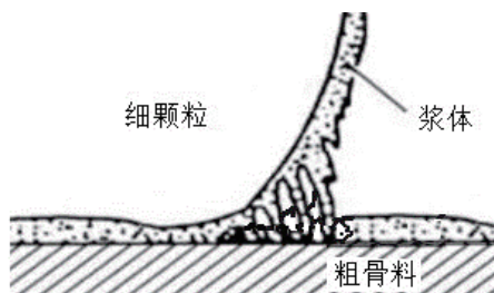
图4 水泥浆体与固体颗粒黏附示意图
