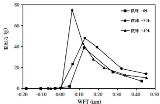
图5 不同微珠掺量时砂浆的水膜厚度与黏附力变化曲线
