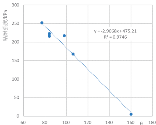
图3 接触角与黏附强度的关系曲线
