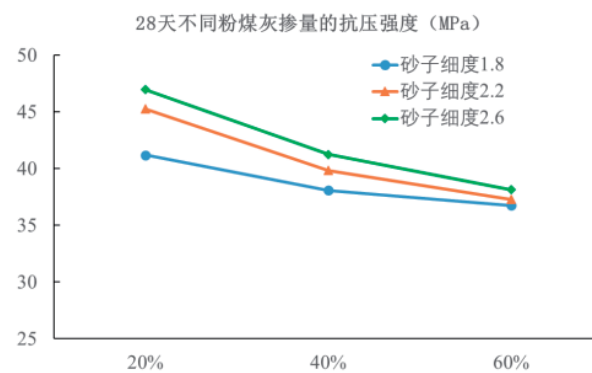
图5 28天不同粉煤灰掺量抗压强度
