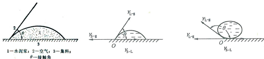
图2 接触角示意图
